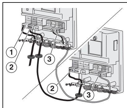
Afb. 4 Twee modules met elkaar verbinden, Netspanning aansluiten
