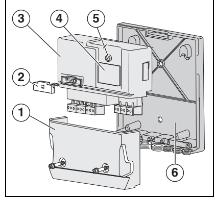
Sekil 1 Genel Bakış EM10
