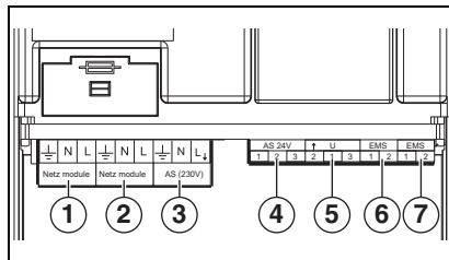
Fig. 2 Conexiones
