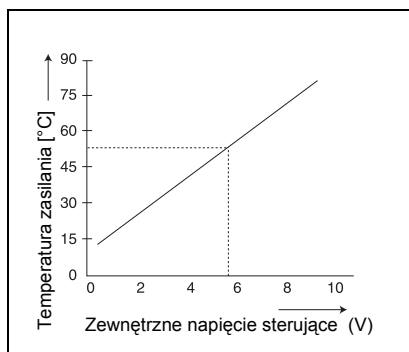
Rys. 3 0-10 V Diagram
