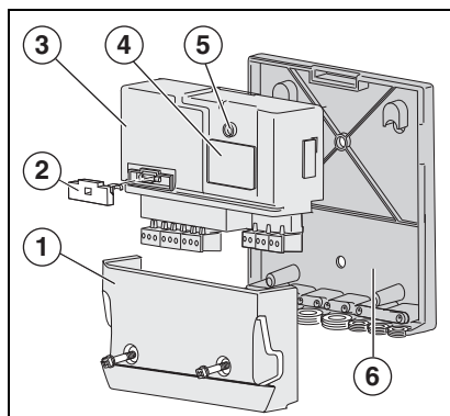
Rys. 1 Rysunek poglądowy
