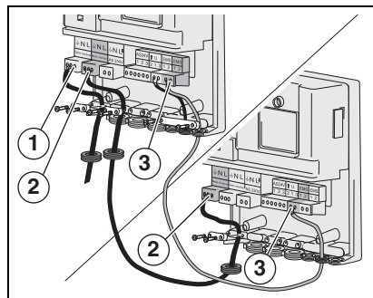
4. ábra Két modul összekötése, a hálózati csatlakozás létrehozása
