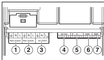
Obr. 2 Připojky
