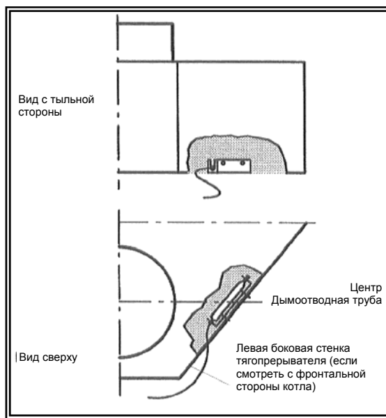
Рис. 10: Датчик температуры дымовых газов на котле G234, типоразмер 7 секций и G334 XZ
