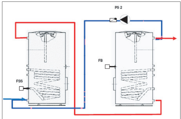
Мал. 4 Циркуляційний насос для перемикання рядів бойлерів
