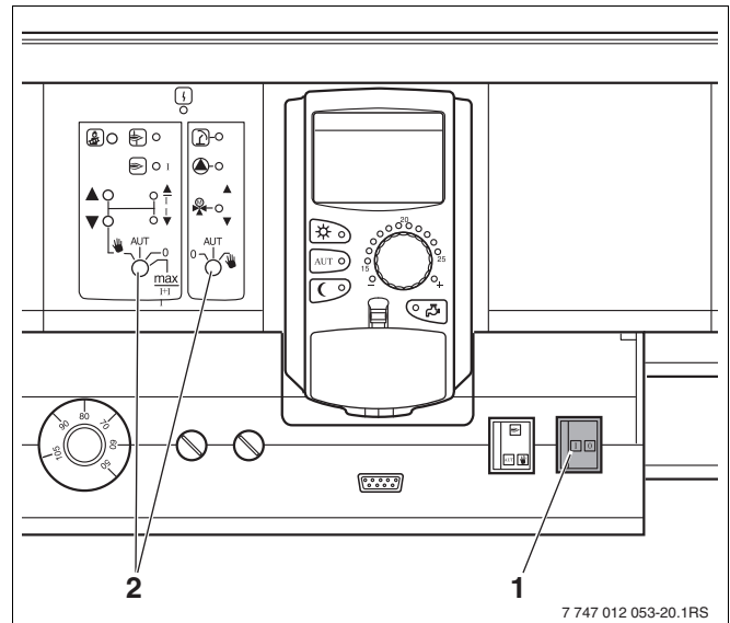
Мал. 8 Робочий вимикач
