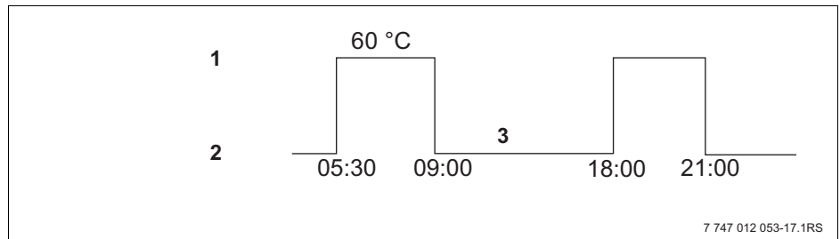
Мал. 10 Приклад: Підігрів гарячої води
