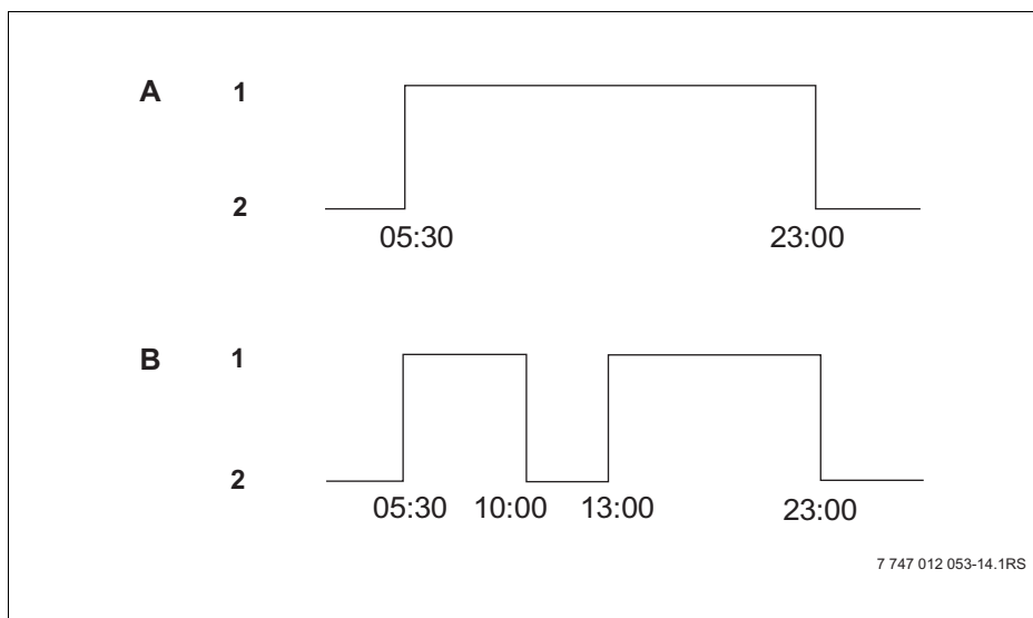
Мал. 16 Уведіть пункти перемикання, щоб призупинити фазу опалення.
