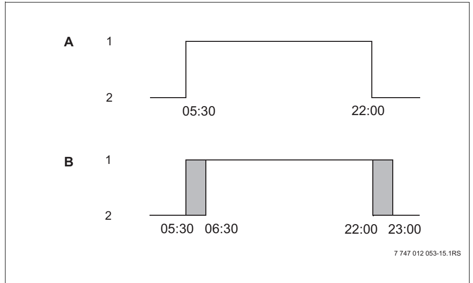
Мал. 14 Змініть період перемикання з 05:30 на 06:30 та з 22:00 на 23:00 (Приклад)
