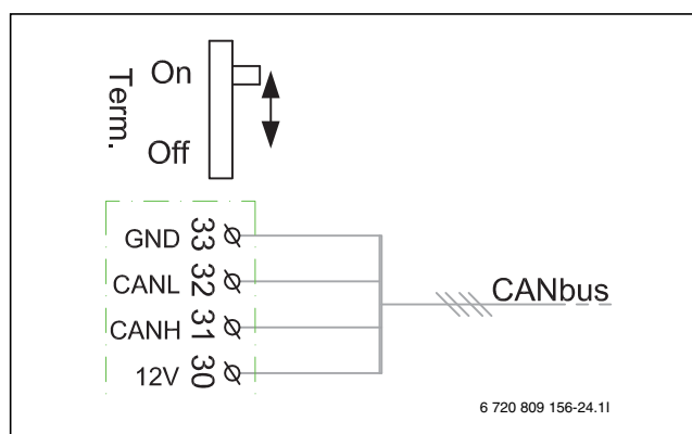
Мал. 13 Термінування CAN-BUS
