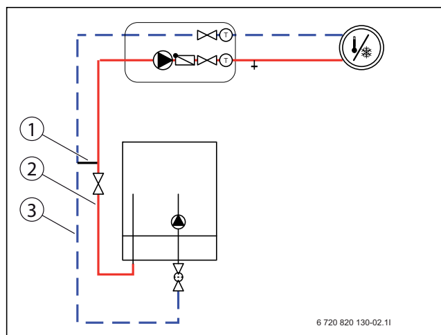
Мал. 3 Внутрішній блок з опалювальним контуром і байпасом
