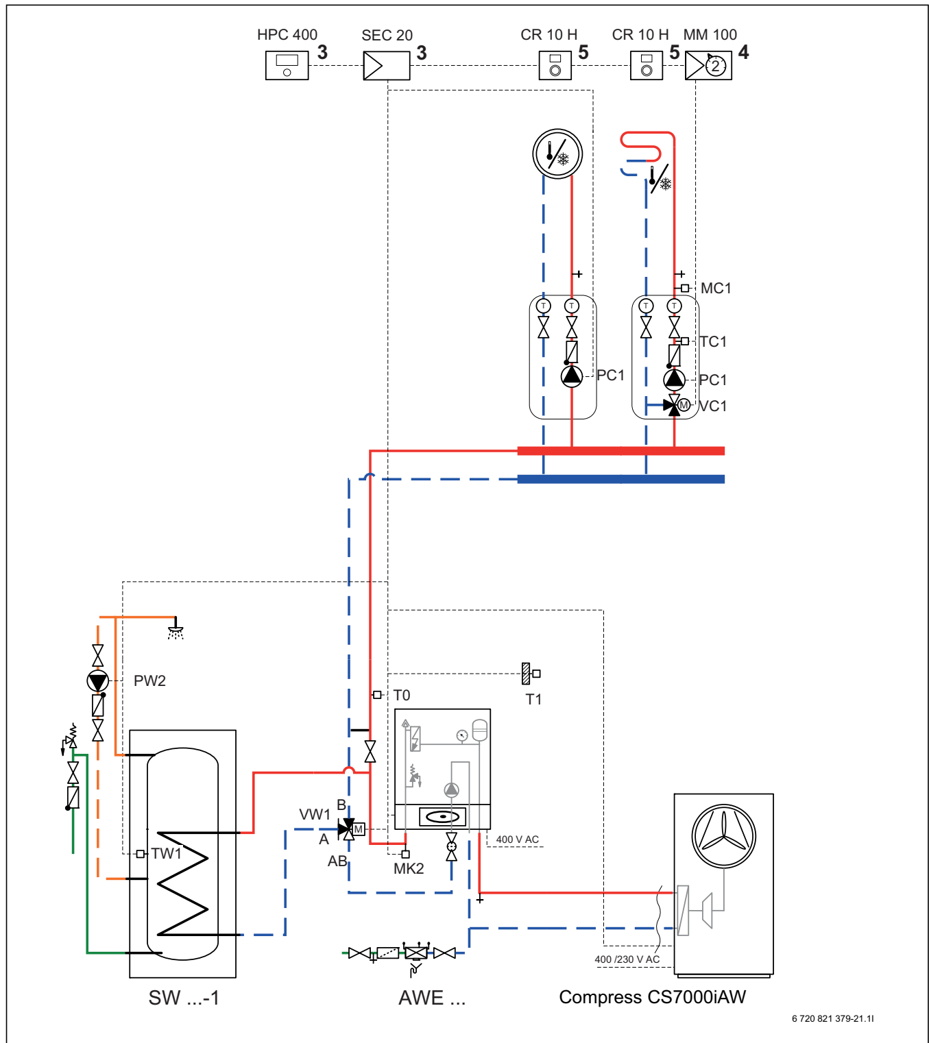
Мал. 8 Додатковий електричний нагрівач із баком непрямого нагріву
