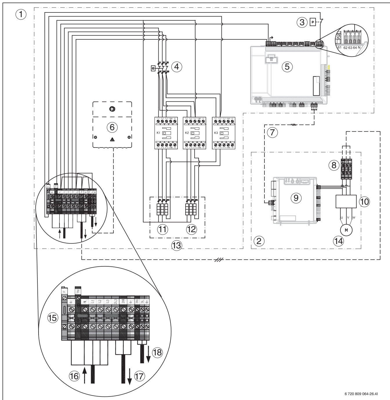
Мал. 39 Однофазний тепловий насос та трифазний вбудований додатковий електричний нагрівач
