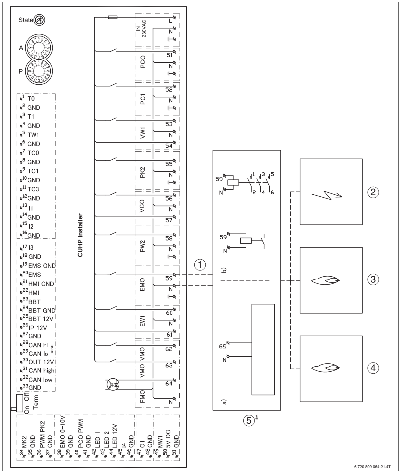
Мал. 24 Схема з'єднань монтажного модуля, пуск/зупинка
