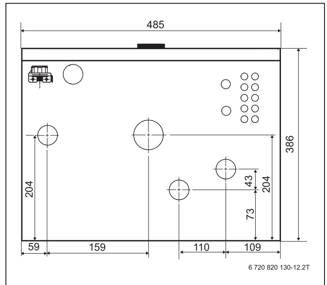
Мал. 31 Внутрішній блок із додатковим електричним нагрівачем AWE, розміри в мм (вигляд знизу)
