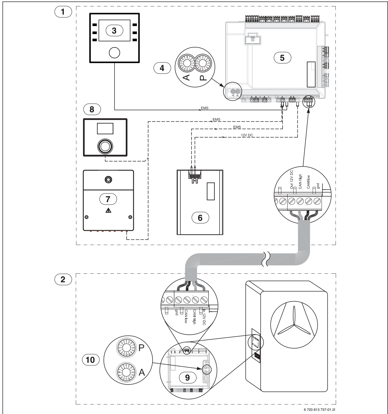
Мал. 27 Внутрішній блок для бівалентної експлуатації – огляд CAN/EMS-BUS
