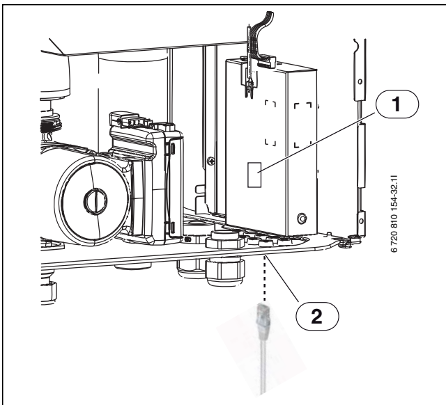
Мал. 44 IP-модуль
