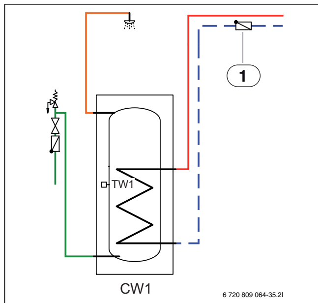
Мал. 46 Водонагрівач
