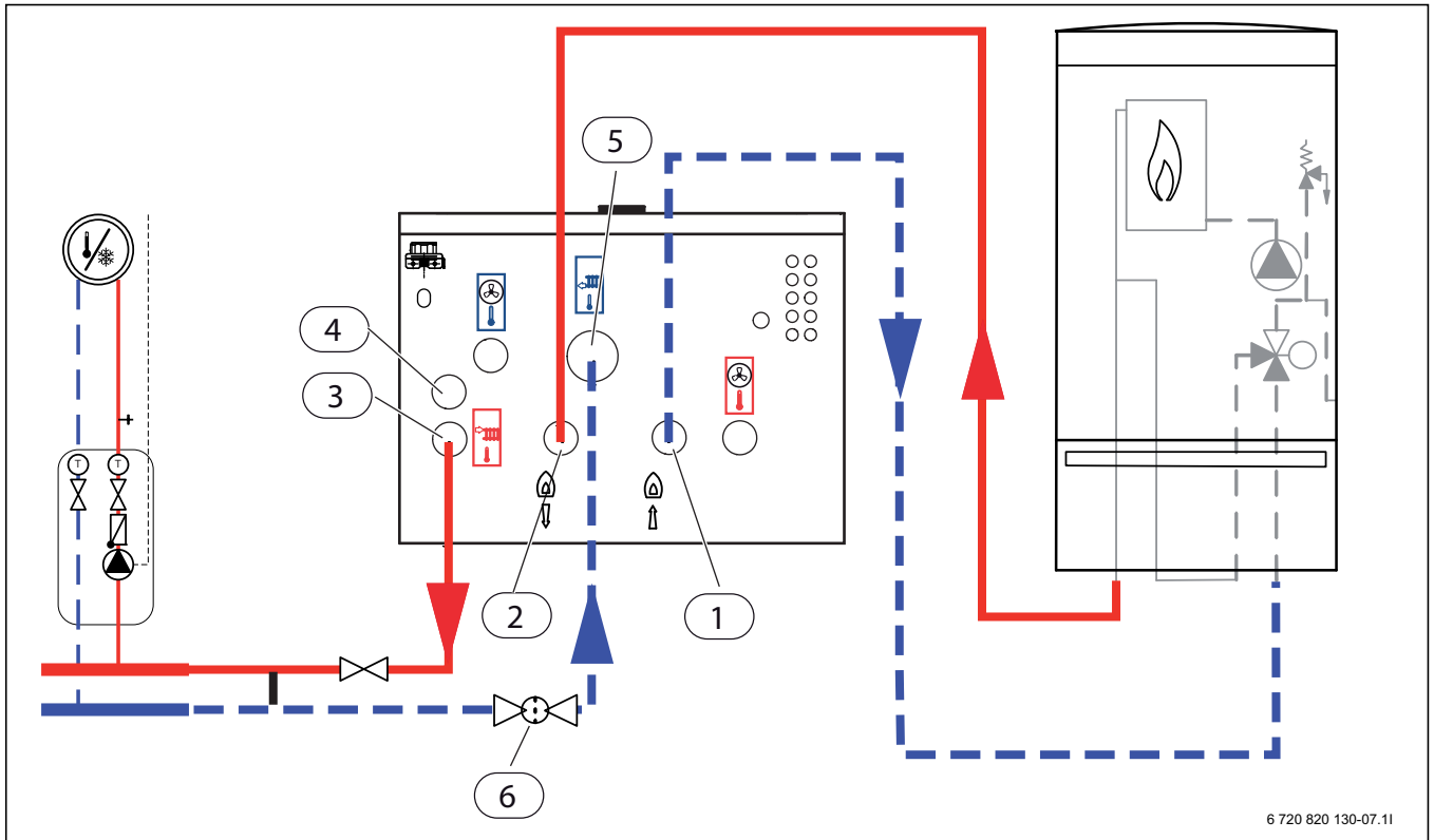
Мал. 20 Підключення внутрішнього блоку для бівалентної експлуатації AWB у системі опалення та додаткового джерела тепла
