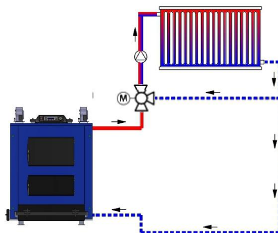
Рис.10 Схема монтажу з якісним регулюванням.
