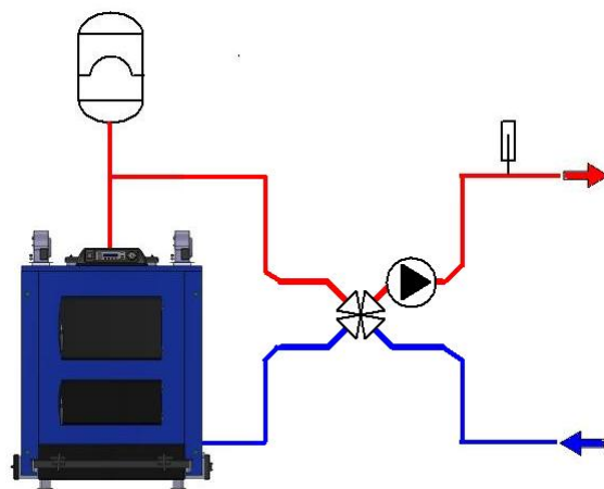
Рис.6 Чотириходовий клапан
