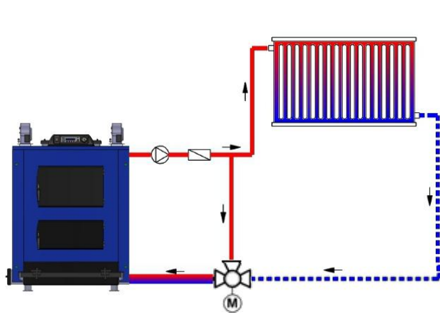
Рис.9 Схема монтажу в захисній конфігурації.
