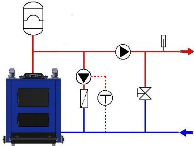
Рис.4 Дозуючо-змішувальний насос
