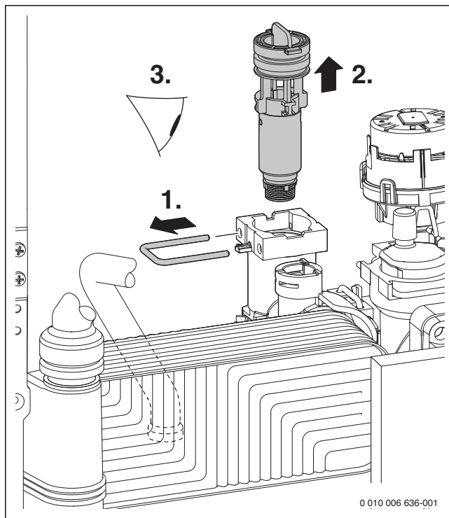
Мал. 51 Перевірка фільтра в трубі холодної води
