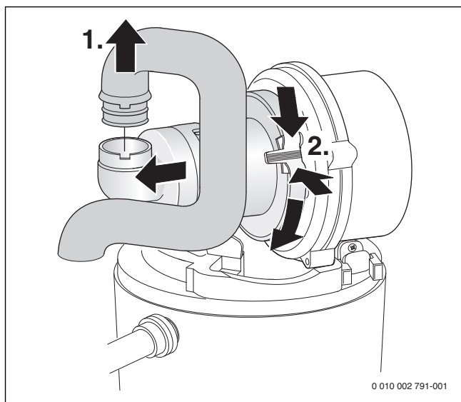
Мал. 40 Демонтаж впускної труби та змішувальної камери
