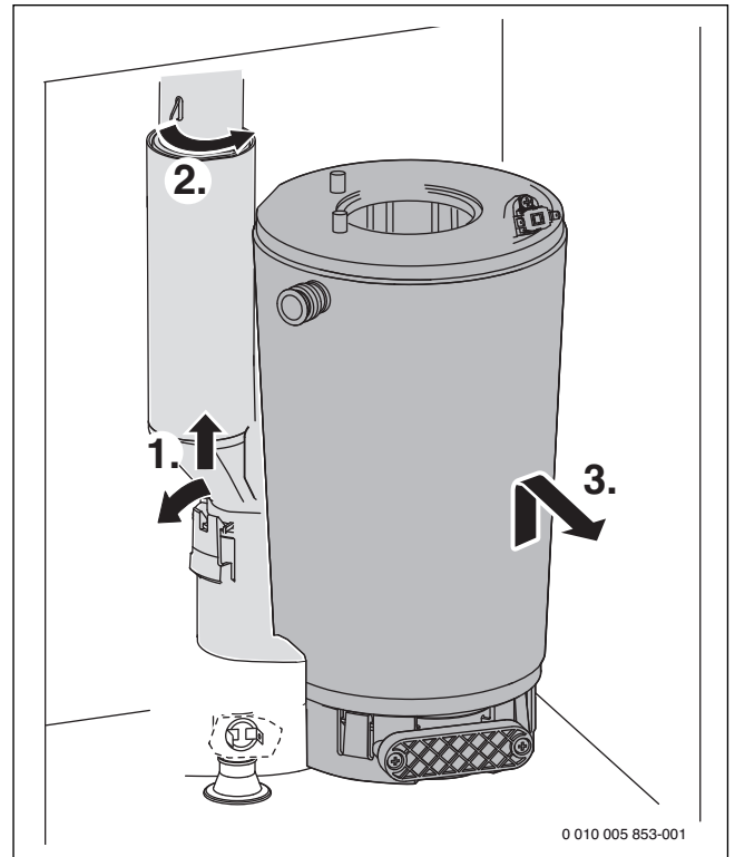
Мал. 60 Демонтаж котлового блока, який включає камеру згоряння і теплообмінник
