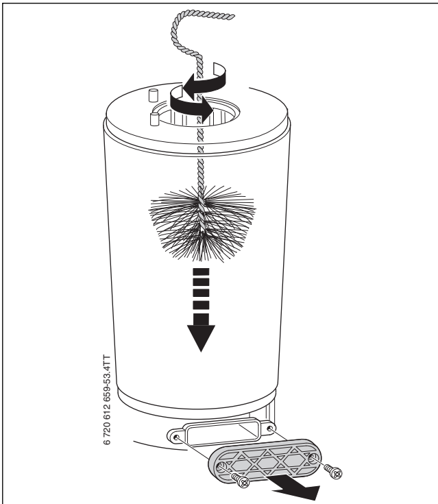
Мал. 45 Чищення теплообмінника
