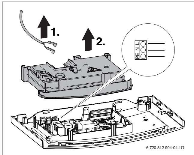
Мал. 27 Заміна мережевого кабелю
