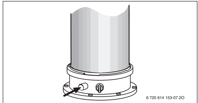
Мал. 34 Штуцер для вимірювання димових газів
