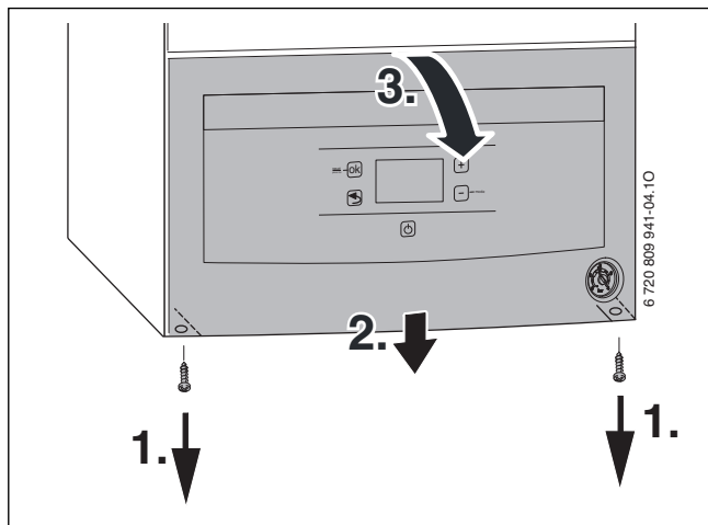
Мал. 21 Відкидання панелі керування вниз
