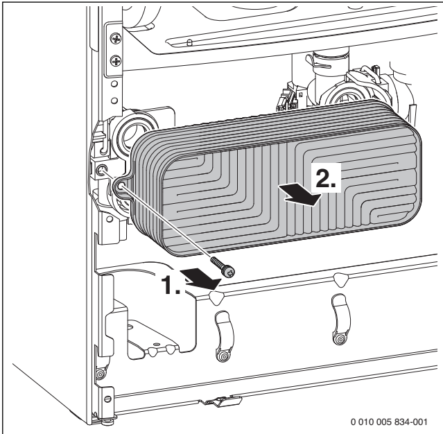
Мал. 52 Демонтаж пластинчастого теплообмінника
