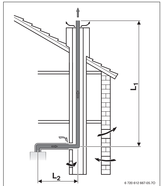
Мал. 8 Відведення димових газів у шахті згідно з B_{33(x)}
