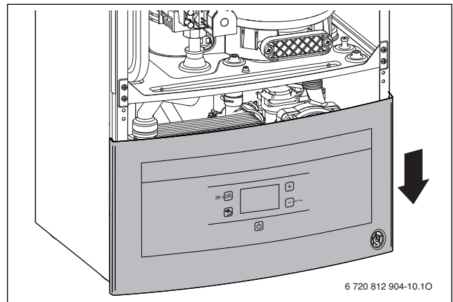
Мал. 33 Панель керування, залишена у рамі для одночасного керування газовою арматурою і панеллю керування
