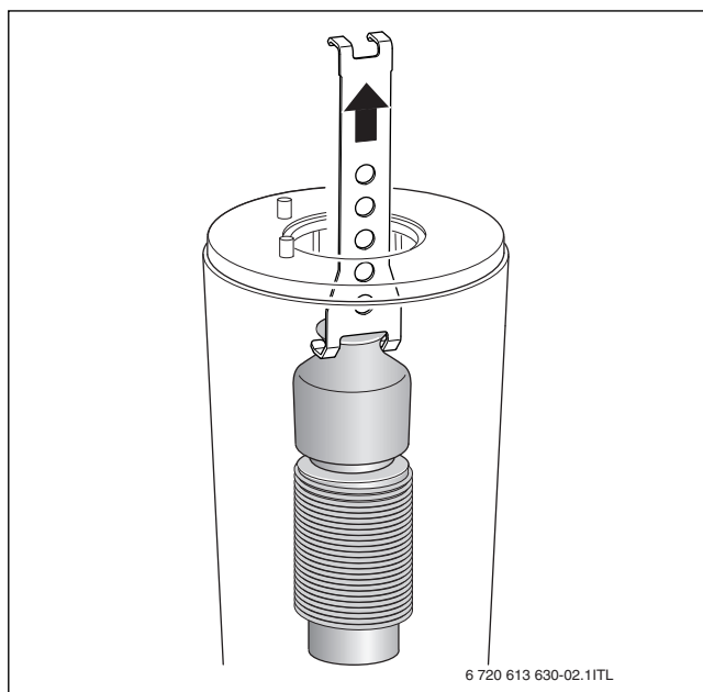
Мал. 43 Виймання верхнього елемента теплообмінника, що служить для оптимізації розподілування тепла
