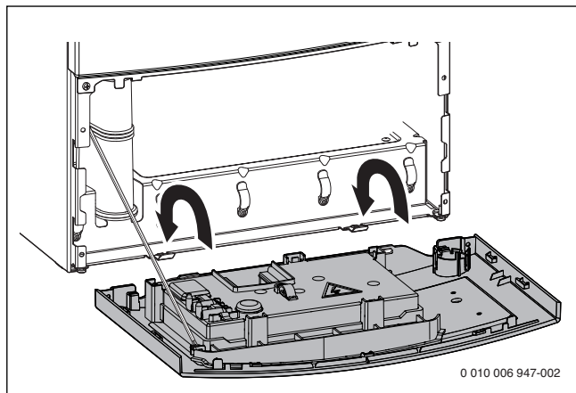
Мал. 22 Встановлення панелі керування у сервісне положення
