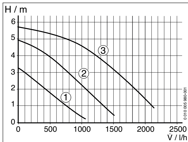
Мал. 32 Характеристична крива насоса опалювального контуру
