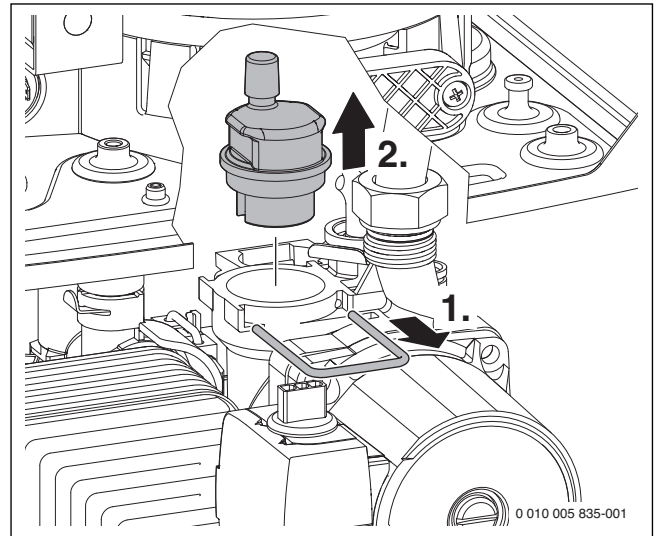
Мал. 53 Демонтаж автоматичного повітровідокремлювача
