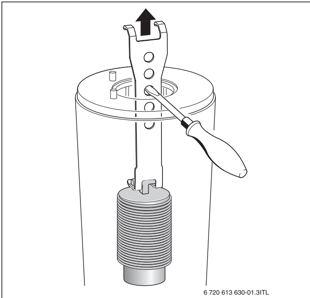
Мал. 44 Виймання нижнього елемента теплообмінника, що служить для оптимізації розподілування тепла
