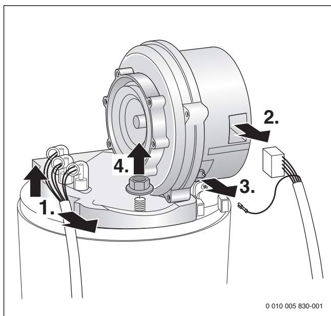
Мал. 41 Виймання вентилятора
