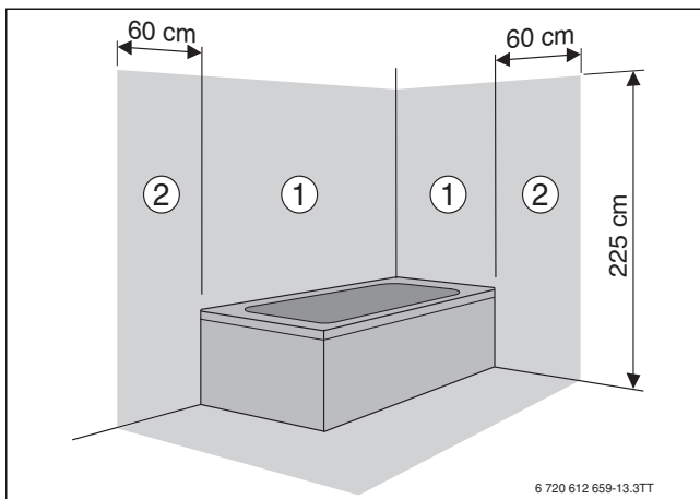
Мал. 25 Зони захисту
