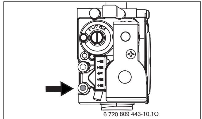
Мал. 37 Штуцер для вимірювання тиску газу
