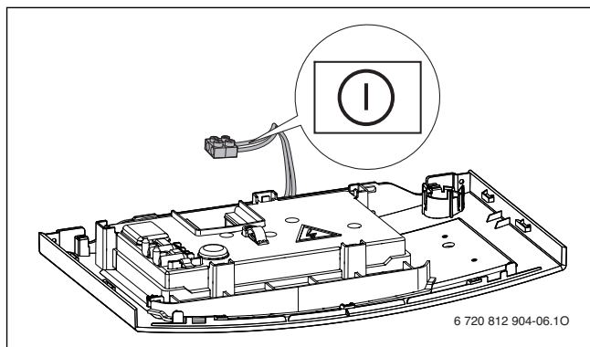
Мал. 28 Зовнішній комутаційний контакт, без потенціалу
