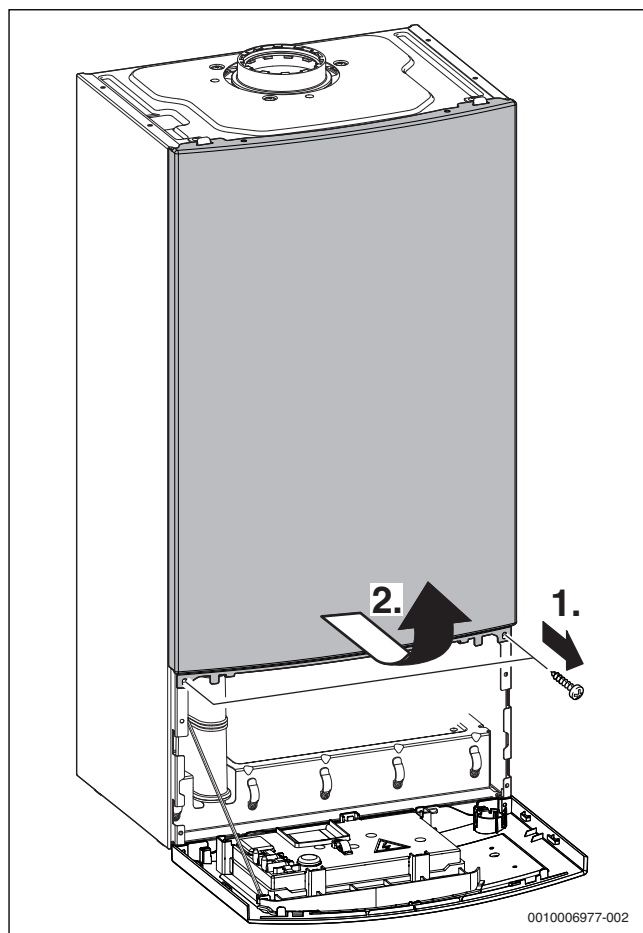
Мал. 23 Демонтаж передньої обшивки
