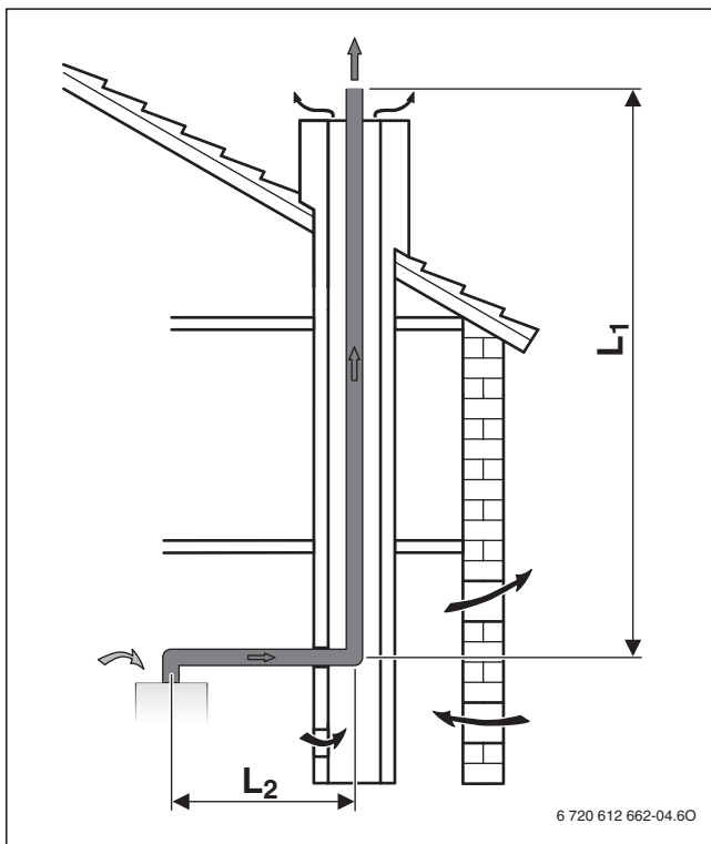
Мал. 7 Відведення димових газів у шахті згідно з B_{23}
