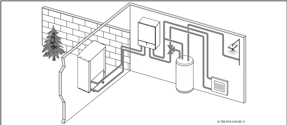
Мал. 2 Тепловий насос CS7000i AW, внутрішній блок теплового насоса AWE з інтегрованим додатковим електричним нагрівачем, зовнішній бак непрямого нагріву
