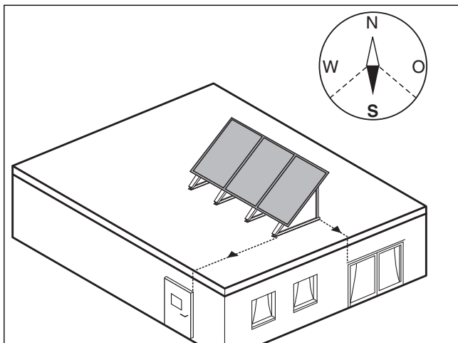
Рис. 10 Розташування колектора
