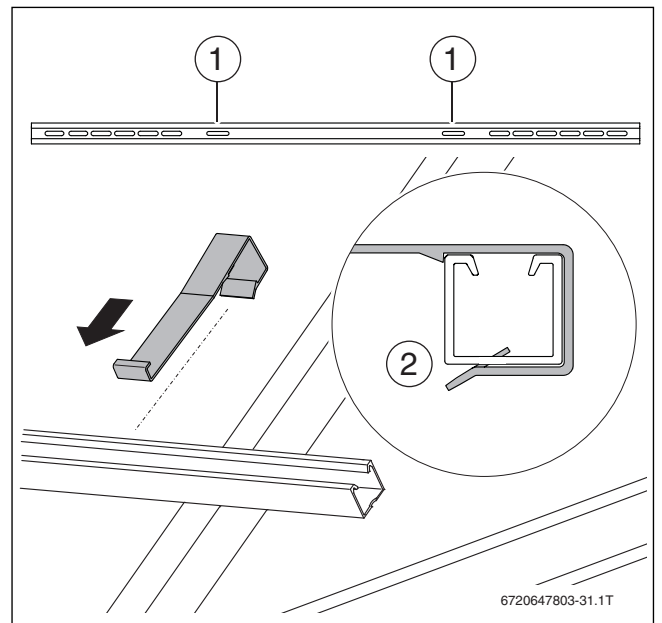
Рис. 49 Монтаж захисту від сповзання
