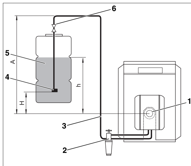
Рис. 37 Топливный бак установлен выше топливного насоса
