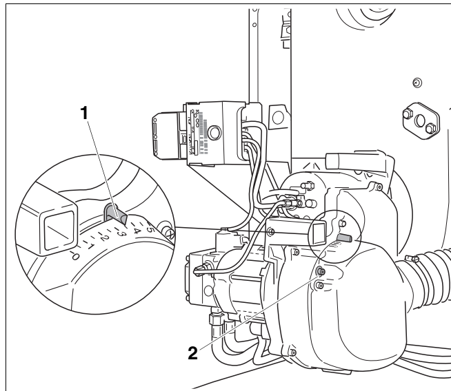
Рис. 17 Проверка положения подвода всасываемого воздуха (ALF)
